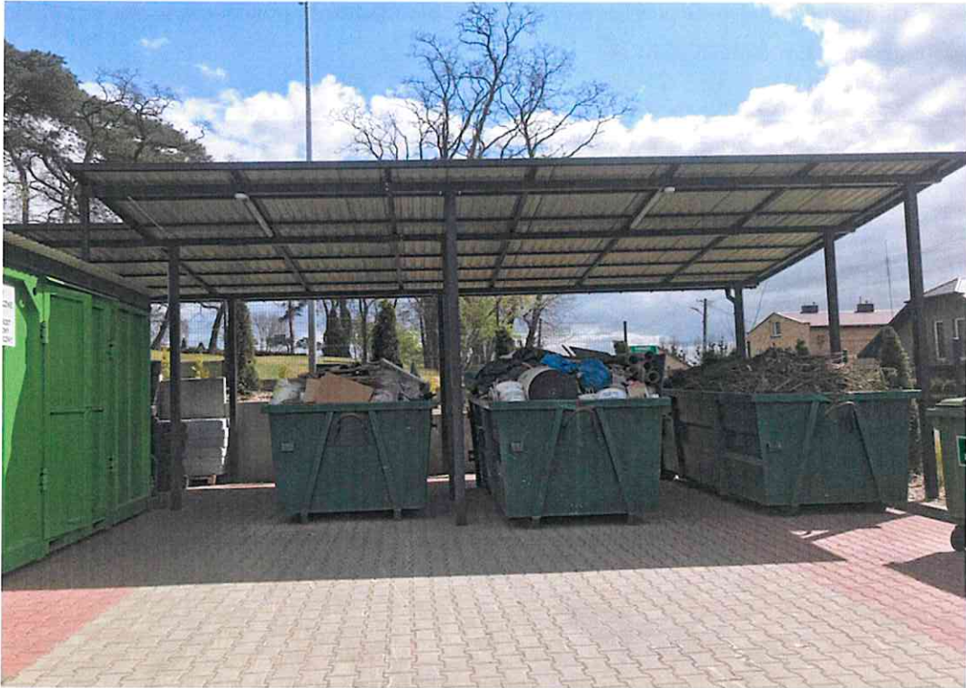
Fot.1 Zadaszenie nad kontenerami w PSZOK w Słupnie
