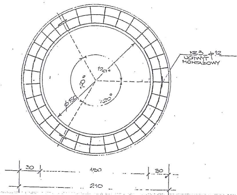
PIERŚCIEŃ ODCIĄŻAJĄCY \phi 2100 \times 1500 SKALA 1:20
