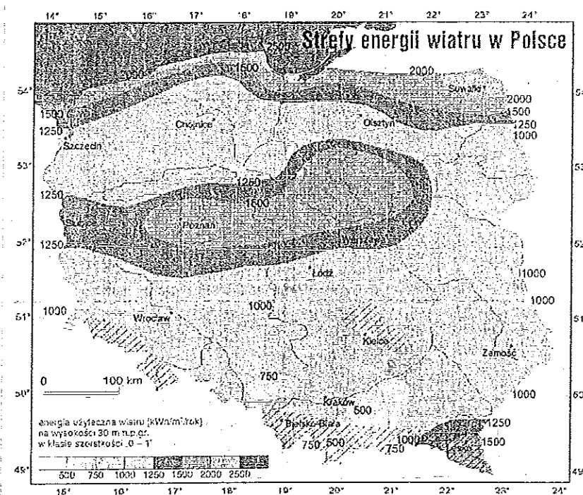
Rysunek 9. Energia użyteczna wiatru w Polsce
