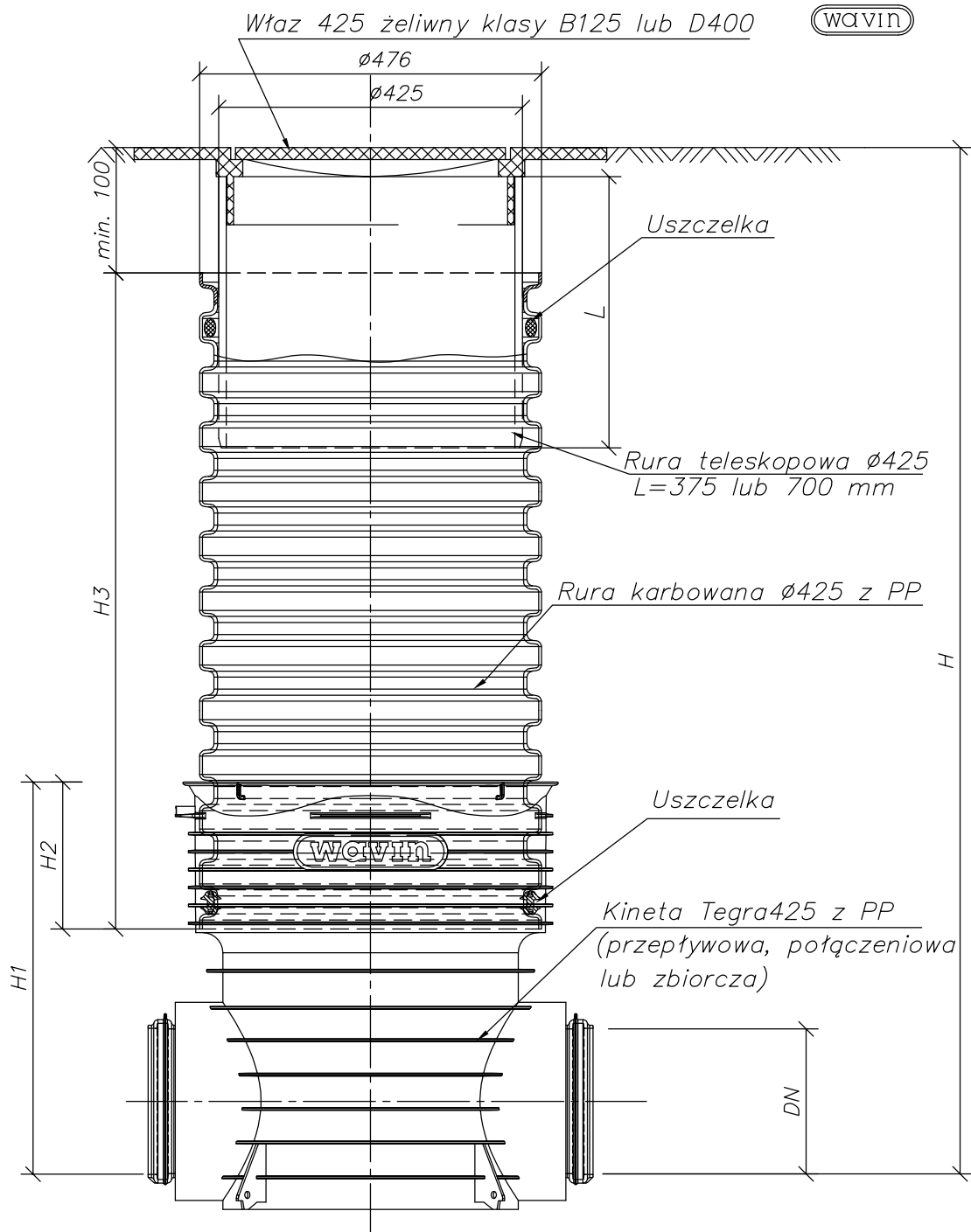
Studzienka inspekcyjna Tegra 425 z rurą teleskopową i włazem żeliwnym klasy B125 lub D400
