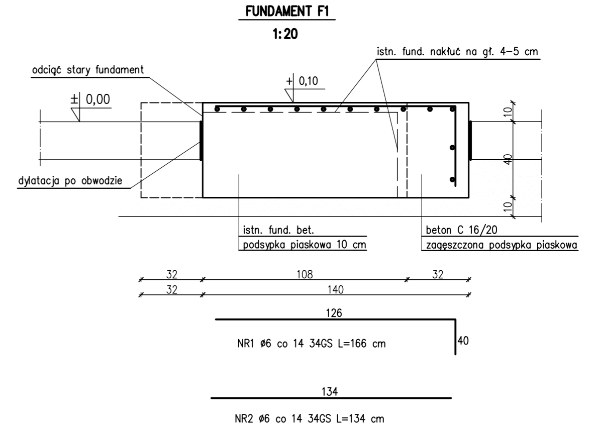
Fundament F2 i F3 w/g opisu
